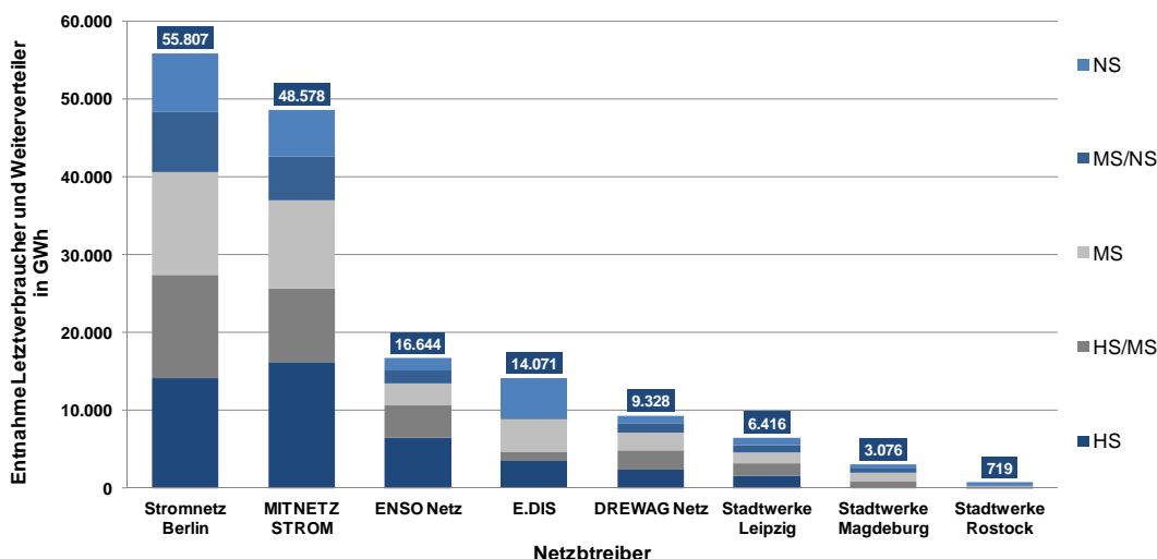
Abbildung 16: Entnahme Letztverbraucher und Weiterverteiler aus dem Stromnetz ausgewählter Verteilnetzbetreiber in Berlin/Brandenburg, Mecklenburg-Vorpommern, Sachsen-Anhalt und Sachsen
