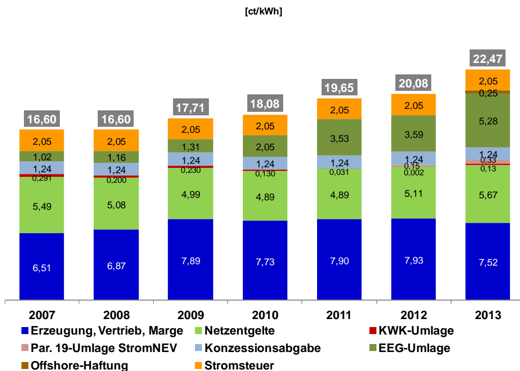
Abbildung 5: Entwicklung des Gewerbestrompreises (durchschnittliches Einzelhandelspreisniveau) und dessen Bestandteile in Deutschland Quelle: [BNetzA 2013] ohne Umsatzsteuer Darstellung und Berechnung: IE Leipzig
