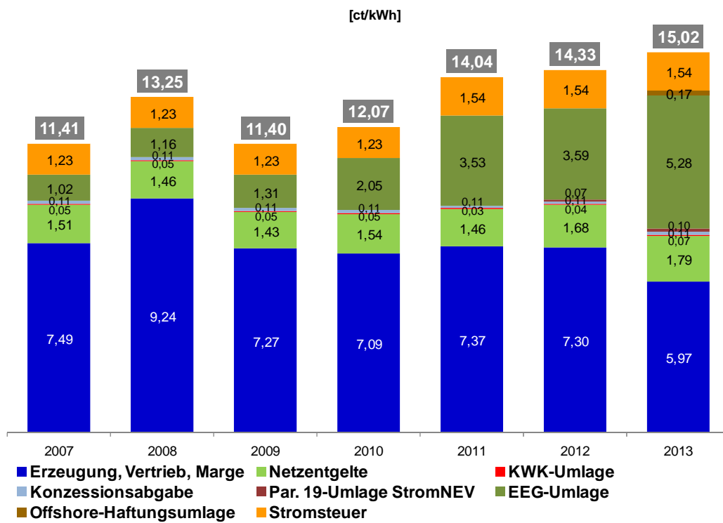
Abbildung 7: Entwicklung des Industriestrompreises und dessen Bestandteile in Deutschland
