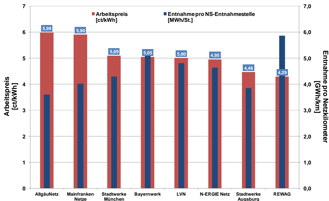
Abbildung 26: Arbeitspreis und Entnahme pro Netzkilometer ausgewählter Verteilnetzbetreiber in Bayern an der Niederspannungsebene
