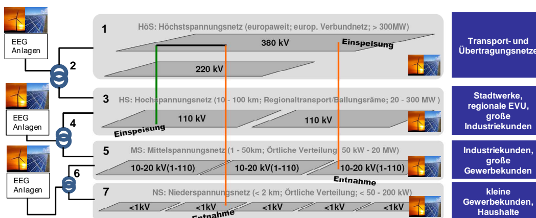
Abbildung 29: Darstellung der Stromnetzebenen in Deutschland Darstellung: IE-LEipzig
